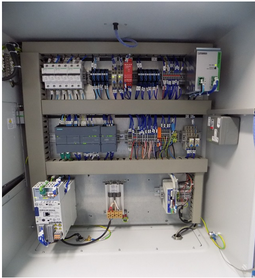
控制柜内部图
